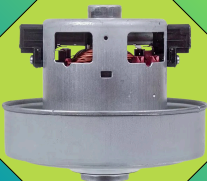
VAM008 SAMSUNG NEW 1400W 220V
